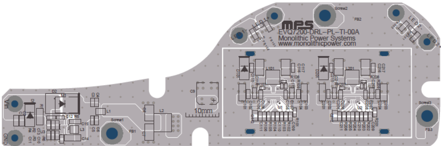
Figure 1—Top Silk & TOP Layer
