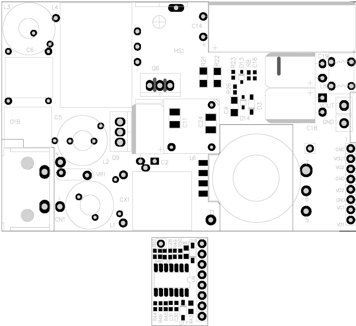
Figure 1—Top Silk Layer
