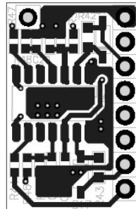
Figure 2—Top Layer
