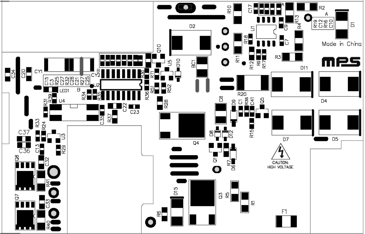
Figure 3—Bottom Silk Layer
