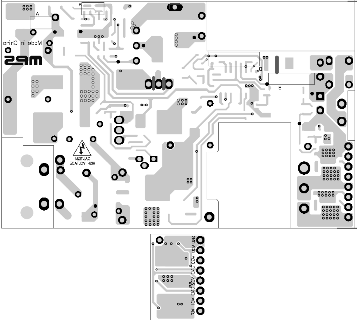
Figure 4—Bottom Layer
